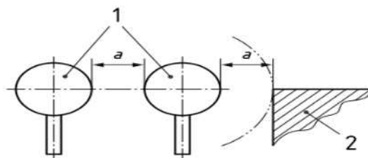
1 수동조작장치, 2 인접부품, a 최소거리
