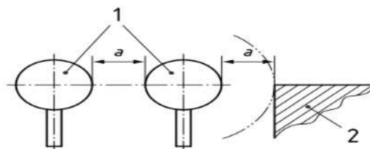
1 수동조작장치, 2 인접부품, a 최소거리
