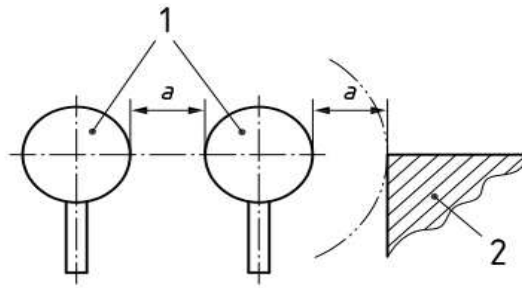
1 수동조작장치, 2 인접부품, a 최소거리
