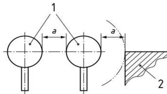
1 수동조작장치, 2 인접부품, a 최소거리
