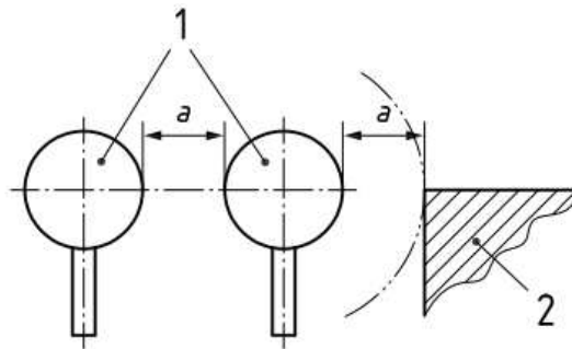
1 수동조작장치, 2 인접부품, a 최소거리
