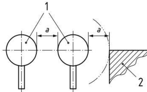
1 수동조작장치, 2 인접부품, a 최소거리
