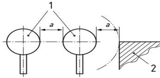
1 수동조작장치, 2 인접부품, a 최소거리
