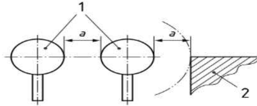
1 수동조작장치, 2 인접부품, a 최소거리
