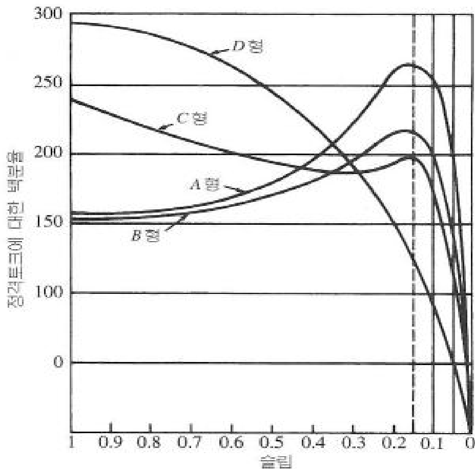
[그림 1] 삼상유도기의 토르크특성 유형
