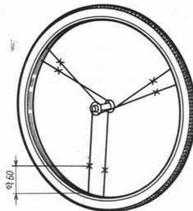
그림 3 스포크 장력
