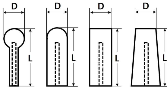
그림 2. 캡의 치수
