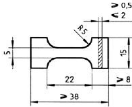
<그림 17> PTFE 시험편
