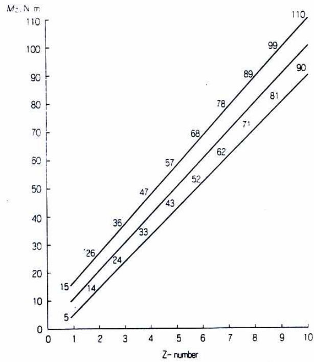
<그림 E.1 M_Z 의 허용오차>
