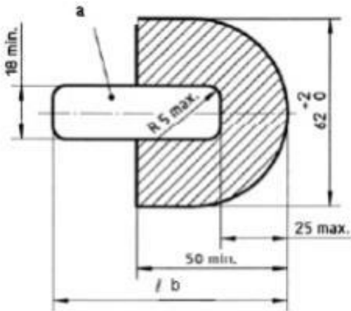
<그림 B.1 관통 시험>
