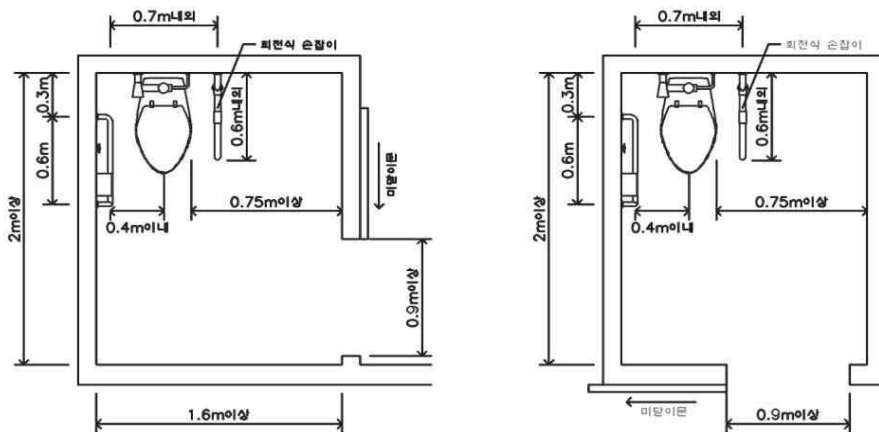
<장애인등의 이용이 가능한 화장실(신축건물)>
