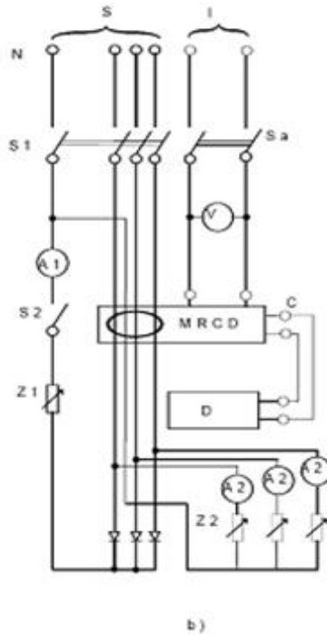
일체형 감지 장치를 가진 MRCD
