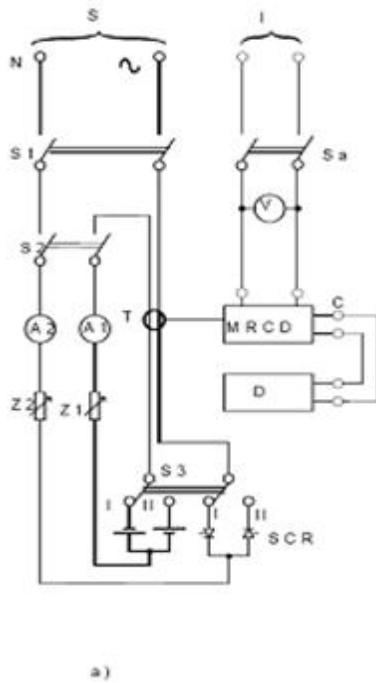
분리형 감지 장치를 가진 MRCD
