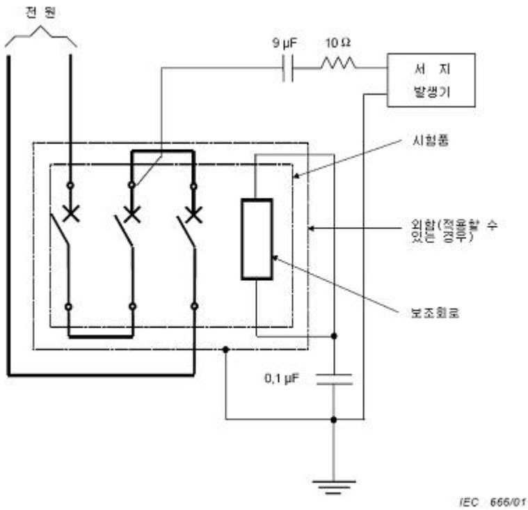
그림 F.10 — F.4.5에 따른 주회로(선-대지간)에서의 서지의 영향을 검증하기 위한 시험회로 - 3극 직렬 접속
