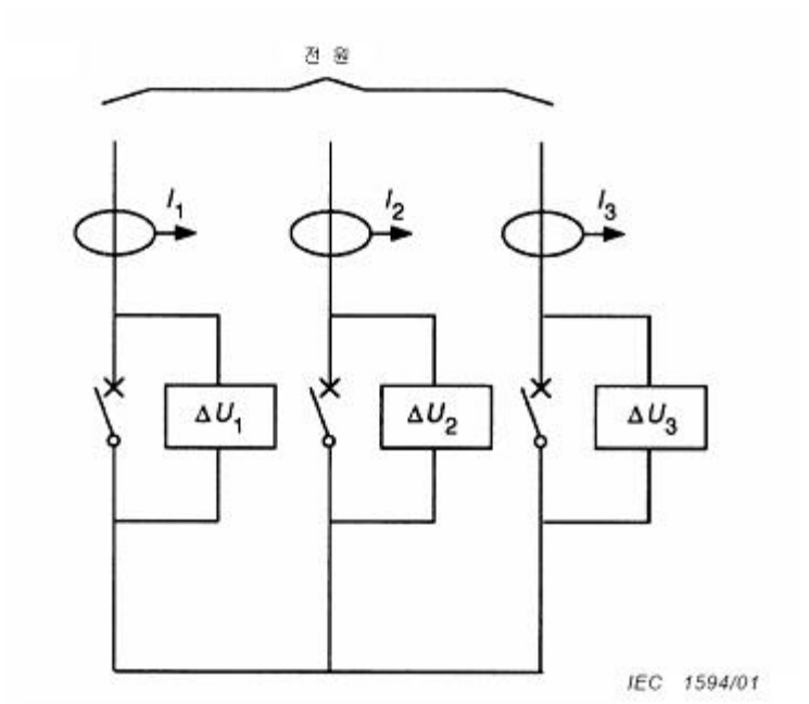
그림 G.1 — G.2.1에 따른 전력손실 측정 예
