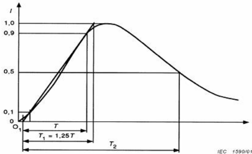
그림 B.6 — 8/20 \mu s 서지 전류 파형
