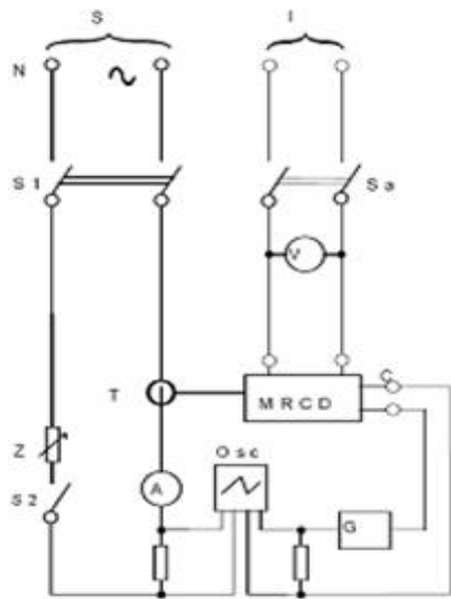
분리형 감지 장치를 가진 MRCD
