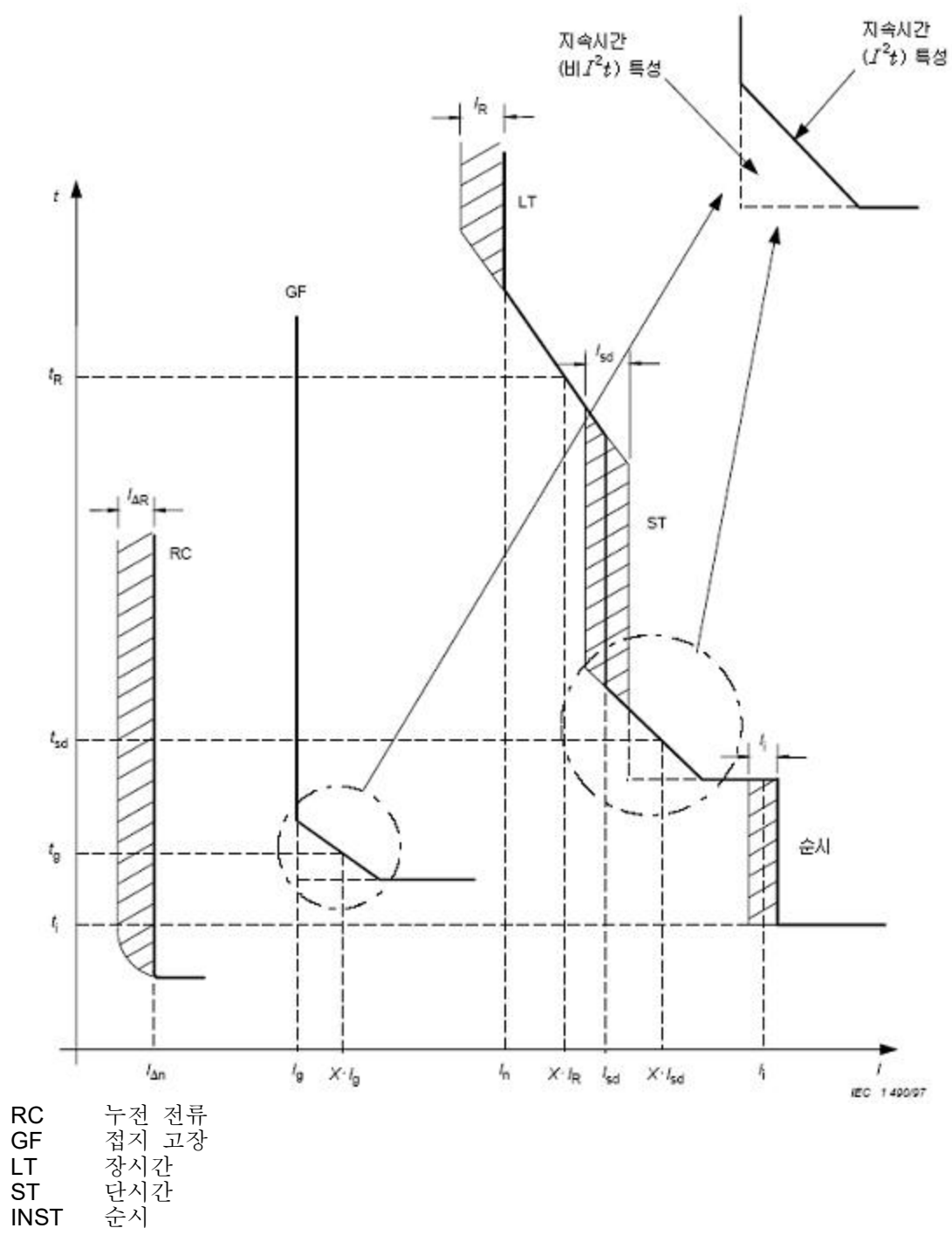
그림 K.1 — 기호와 트립 특성과의 관계
