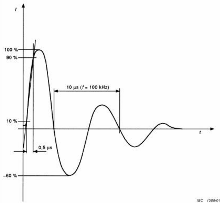
그림 B.4 — 0.5 \mu\text{s}/100 \text{ kHz} 링 웨이브 전류
