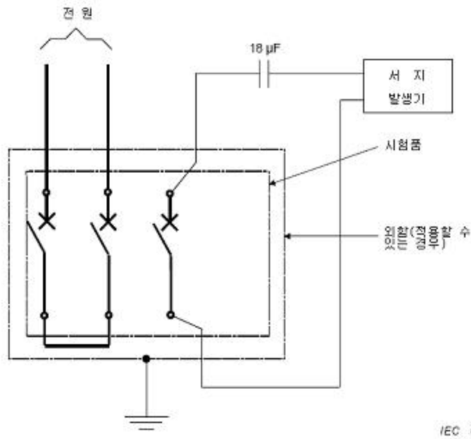
그림 F.12 — F.4.5에 따른 주회로에서의 전류 서지의 영향을 검증하기 위한 시험회로 — 2극 직렬 접속
