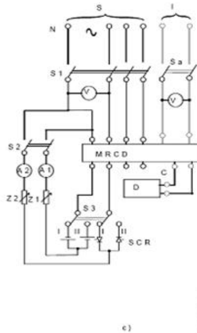
단자형 MRCD
