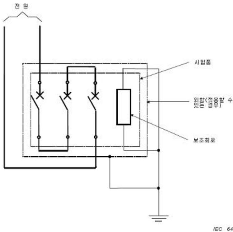
그림 F.3 — F.4.1.3, F.4.2, F.4.3, F.4.6, F.4.7.1, F.5.4, 및 F.6.2에 따른 전자기 내성 및 방사 시험을 위한 시험회로 — 3극 직렬 접속
