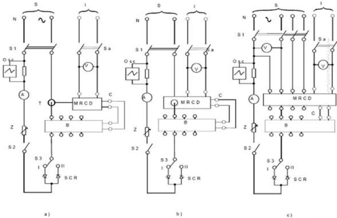
분리형 감지 장치를 가진 MRCD
