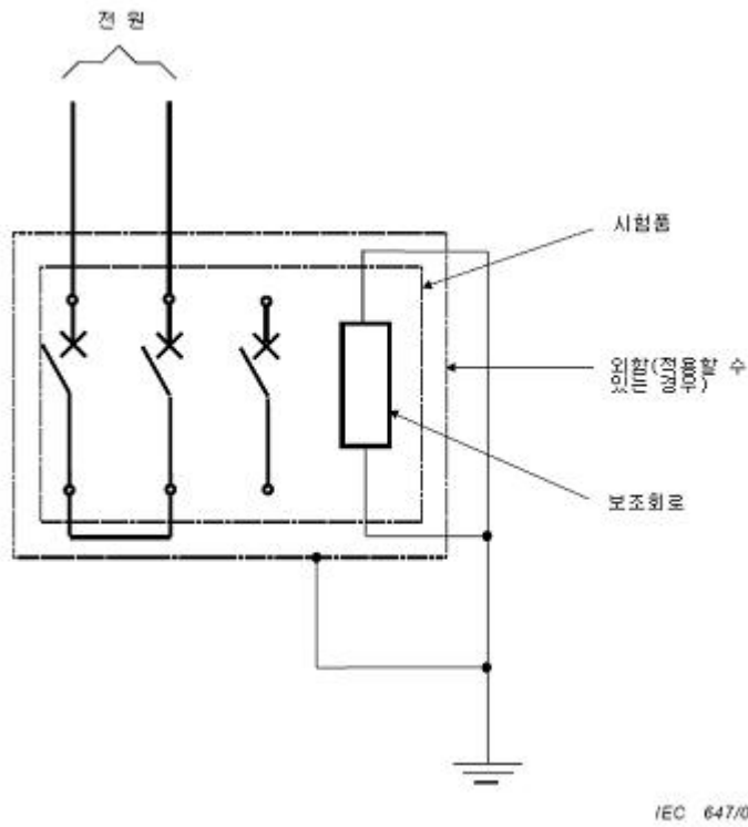
그림 F.2 — F.4.1.3, F.4.2, F.4.3, F.4.6, F.4.7.1, F.5.4 및 F.6.2에 따른 전자기 내성 및 방사 시험을 위한 시험회로 — 2극 직렬 접속
