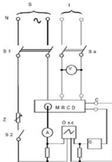
일체형 감지 장치를 가진 MRCD
