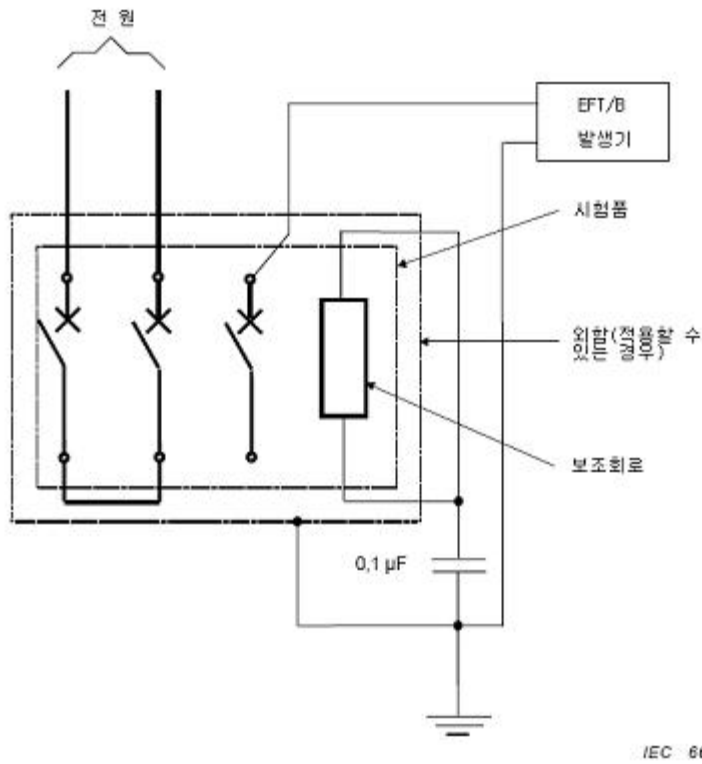
그림 F.6 — F.4.4에 따른 급과도/버스트(EFT/B) 내성 시험회로 - 2극 직렬 접속
