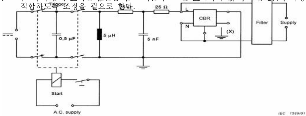
그림 B.5 — 의도하지 않은 트립에 대한 내성 검증을 위한 시험회로의 예
