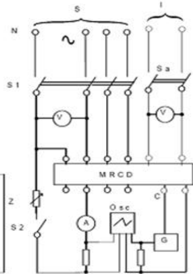
단자형 MRCD
