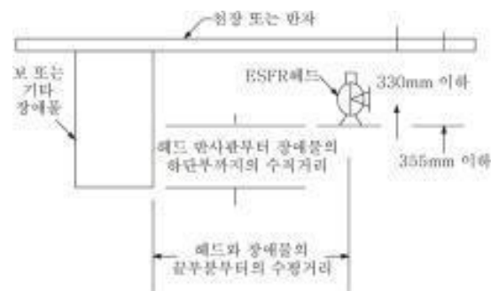
그림 2.7.1.8(1) 보 또는 기타 장애물 위에 head가 설치된 경우의 반사판 위치 (그림 2.7.1.8(3) 또는 표 2.7.1.8(1)을 함께 사용할 것)
