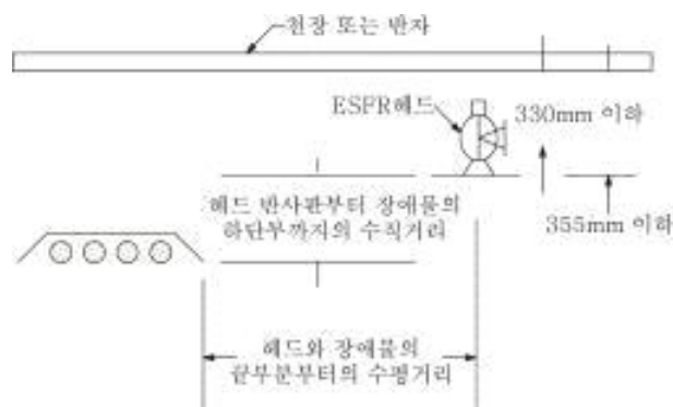
그림 2.7.1.8(2) 장애물이 head 아래에 연속적으로 설치된 경우의 반사판 위치 (그림 2.7.1.8(3) 또는 표 2.7.1.8(1)을 함께 사용할 것)
