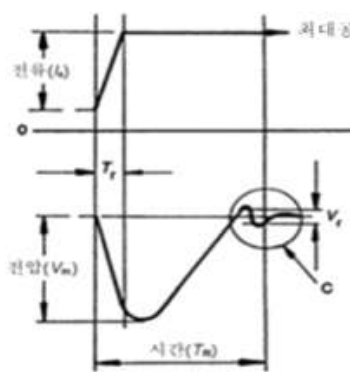
[그림1] : 출력단에 인가된 저항성 부하
