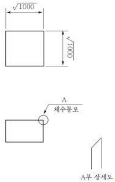
채수통도
