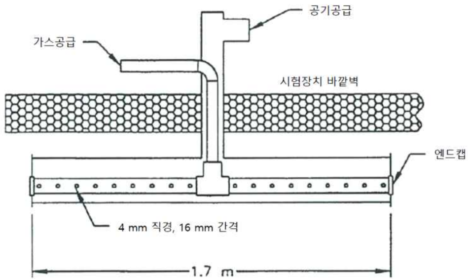
버너 세부도면
