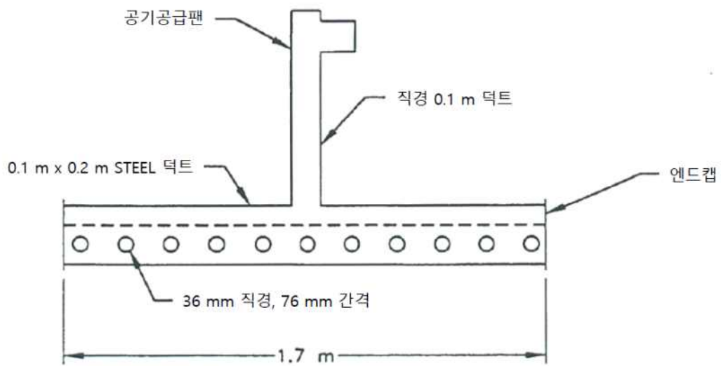
공기공급장치 세부도면
