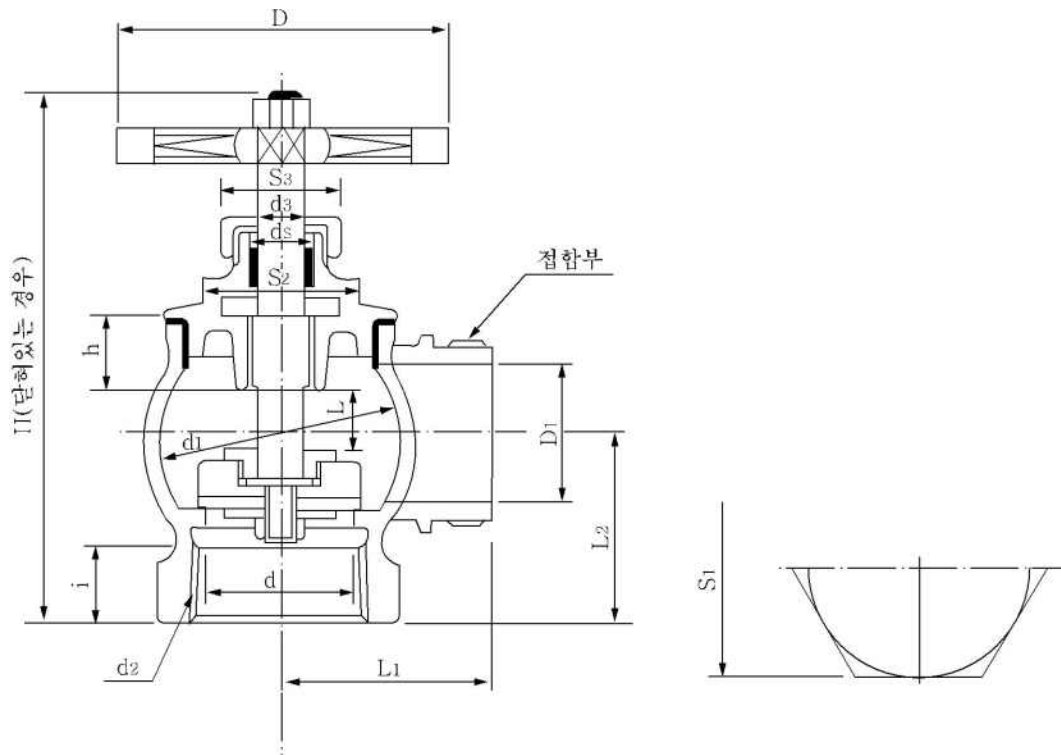
옥내소화전방수구의 구조·모양 및 치수
