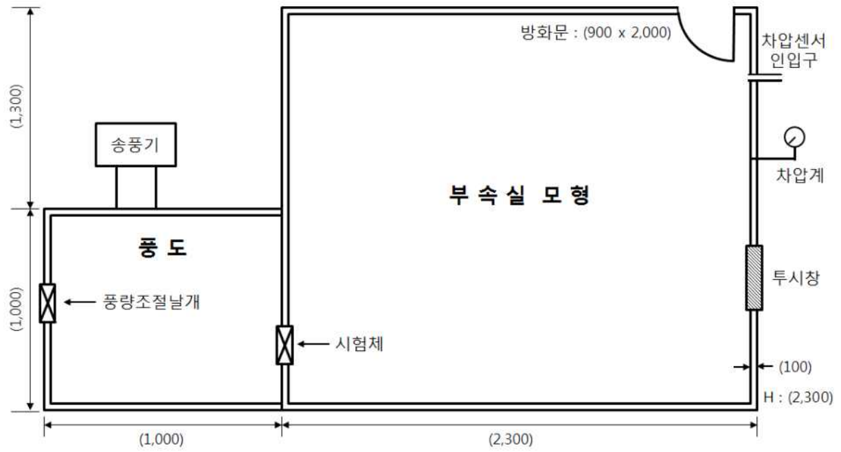
[별표4] 작동시험장치<개정 2018.00.00.>
