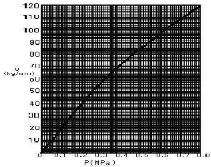
분말헤드의 방사압력 대 방사량곡선
