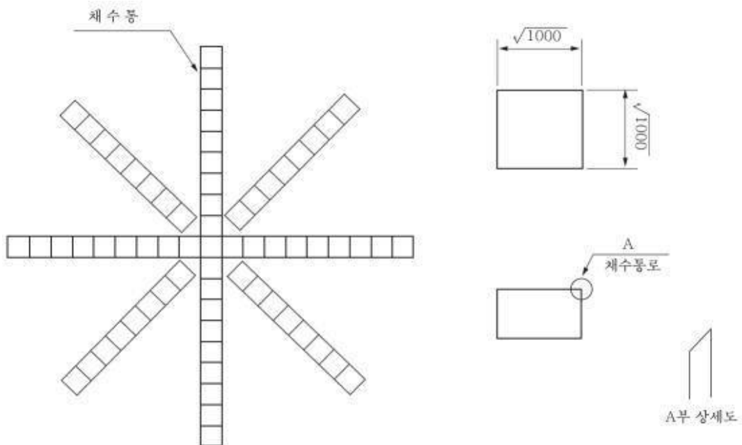
채수통 배치도
