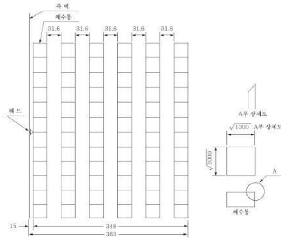
채수통배치도
