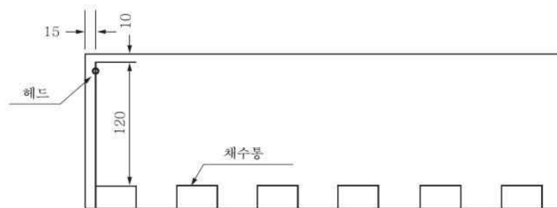
시험장치도
