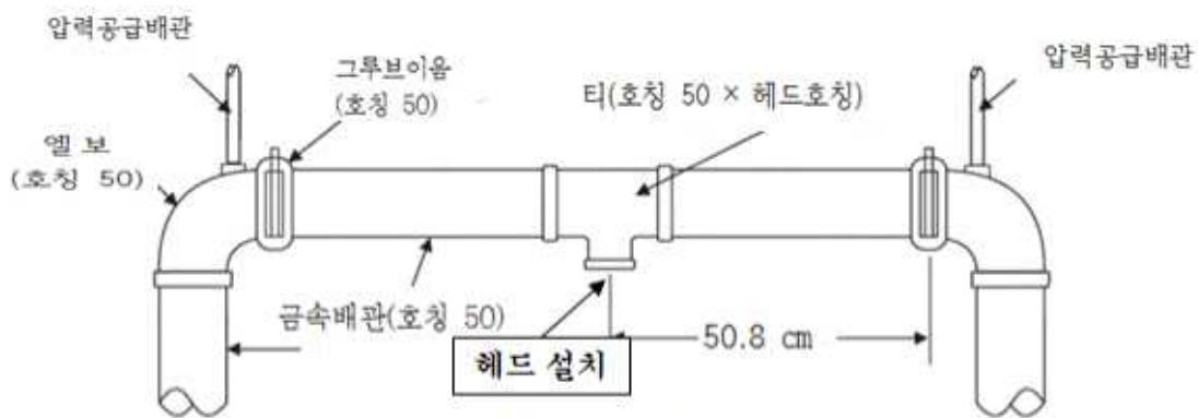
<이중 공급 배관도>
