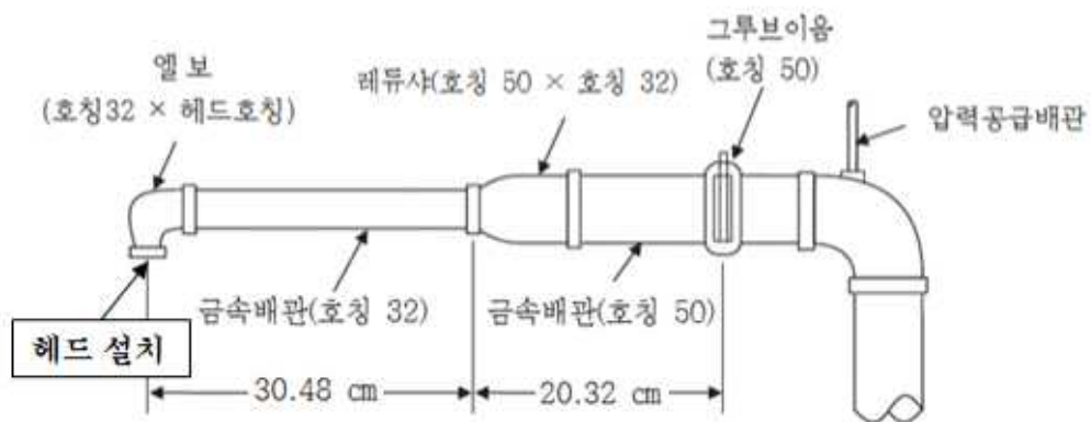
<단일 공급 배관도>
