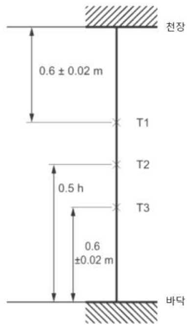
측면도
