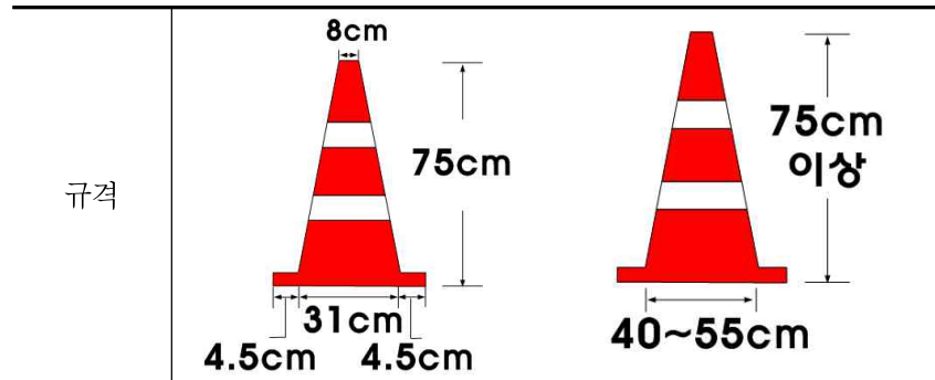
<그림 1.1> 교통콘 규격
