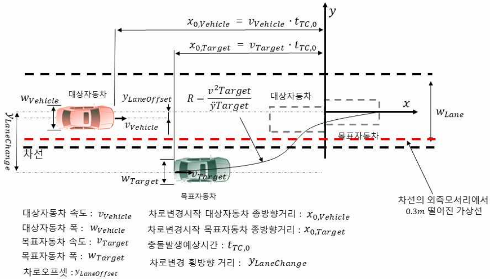
[차로변경 끼어들기 개략도]
