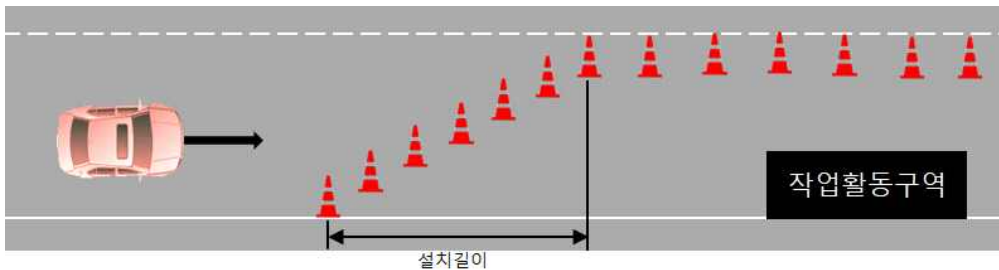
<그림 3.1> 완화구간 설치범위
