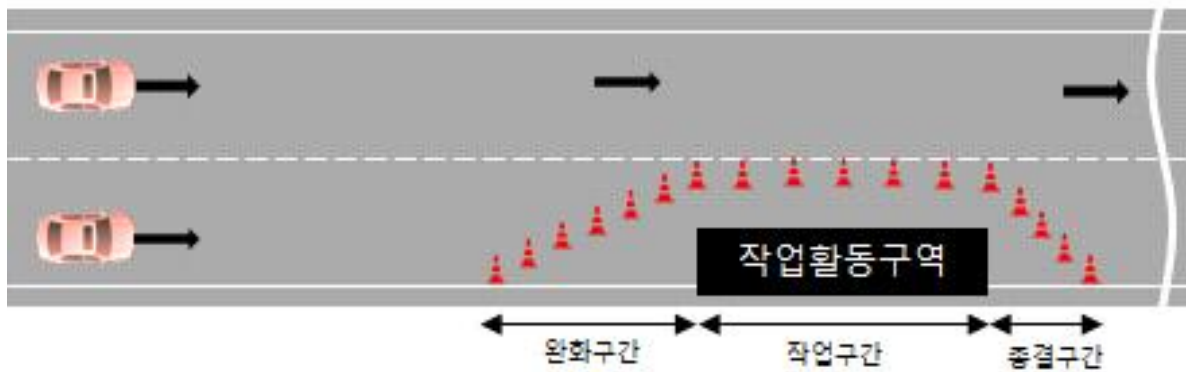
<그림 2.1> 차로 완전 차단
