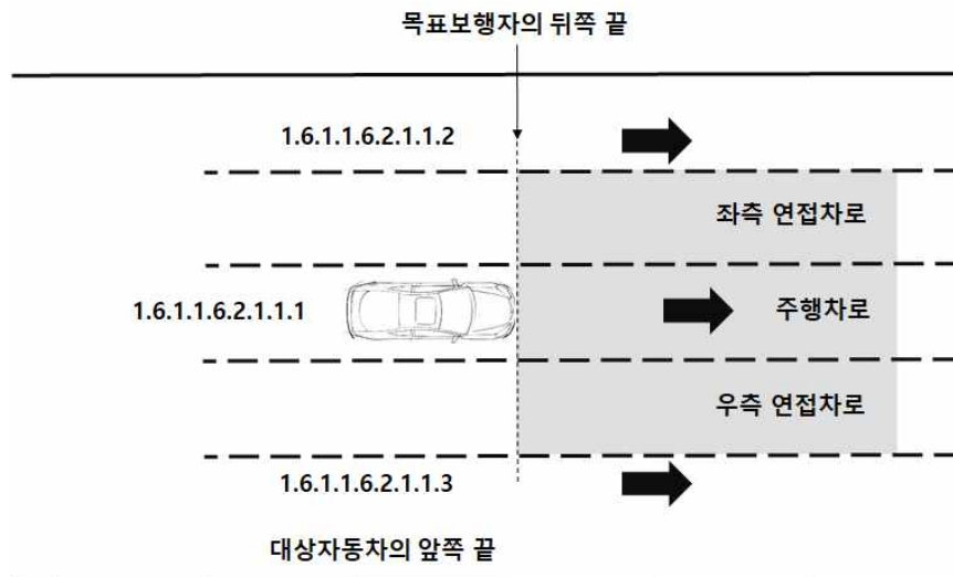
[기타 도로이용자 감지거리 확인시험 개략도]
