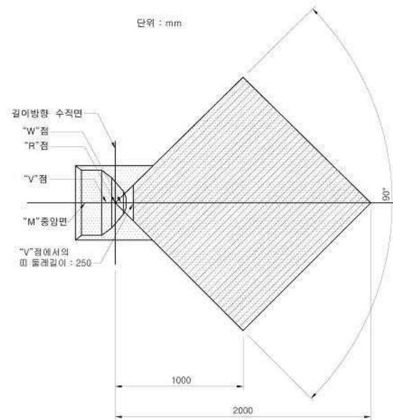
평면의 설치범위도
