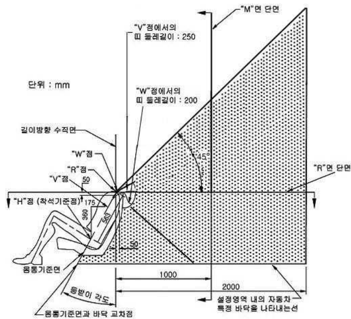
측면의 설치범위도
