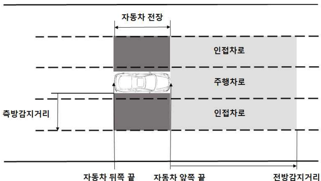
[부분 자율주행시스템의 감지범위]
