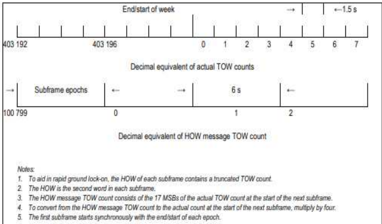
그림 B-5. HOW의 타임라인 관계
