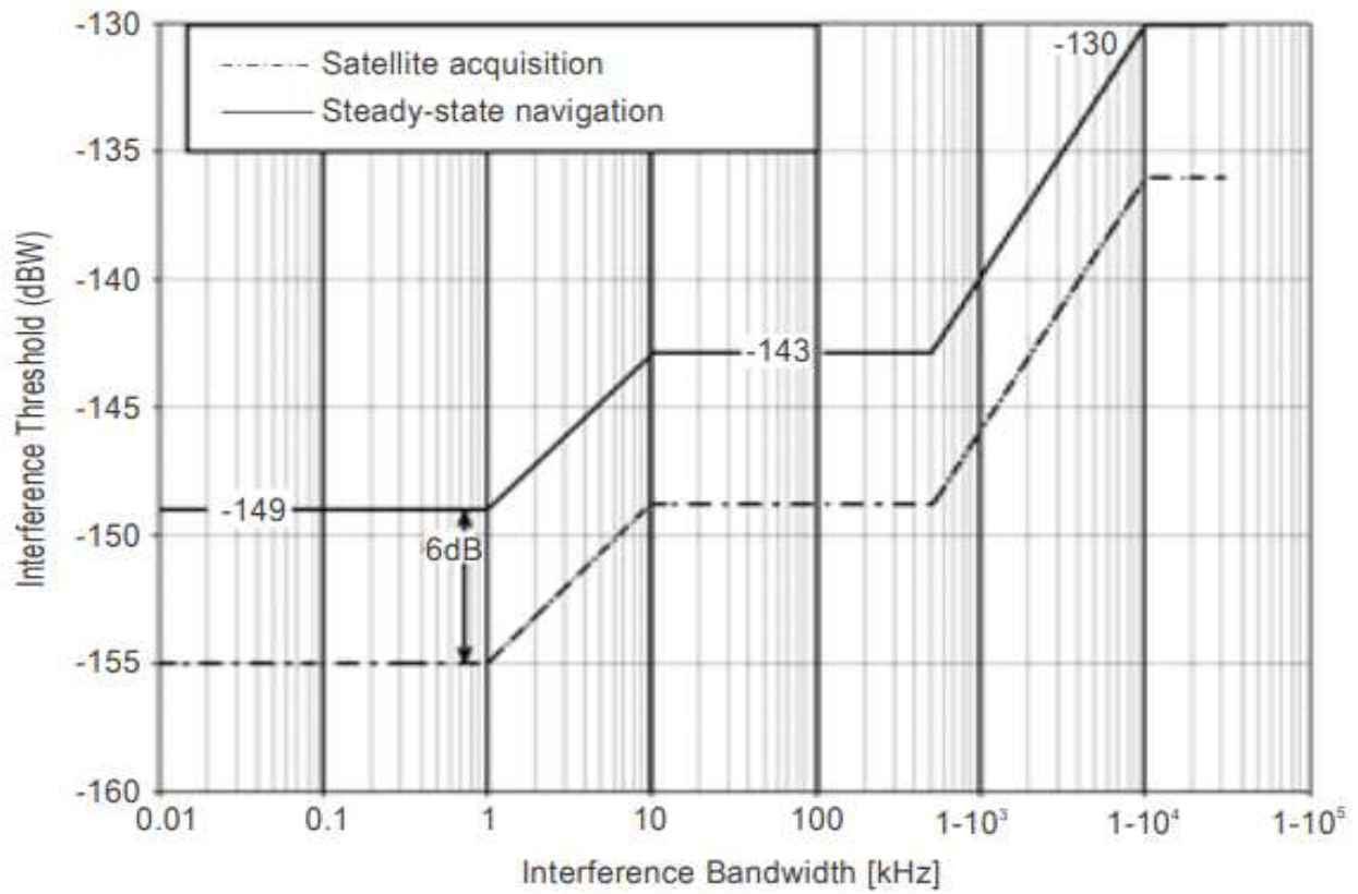
그림 B-38. L1 대역의 GLONASS FDMA 신호 수신기에 대한 간섭 임계값 대 대역폭
