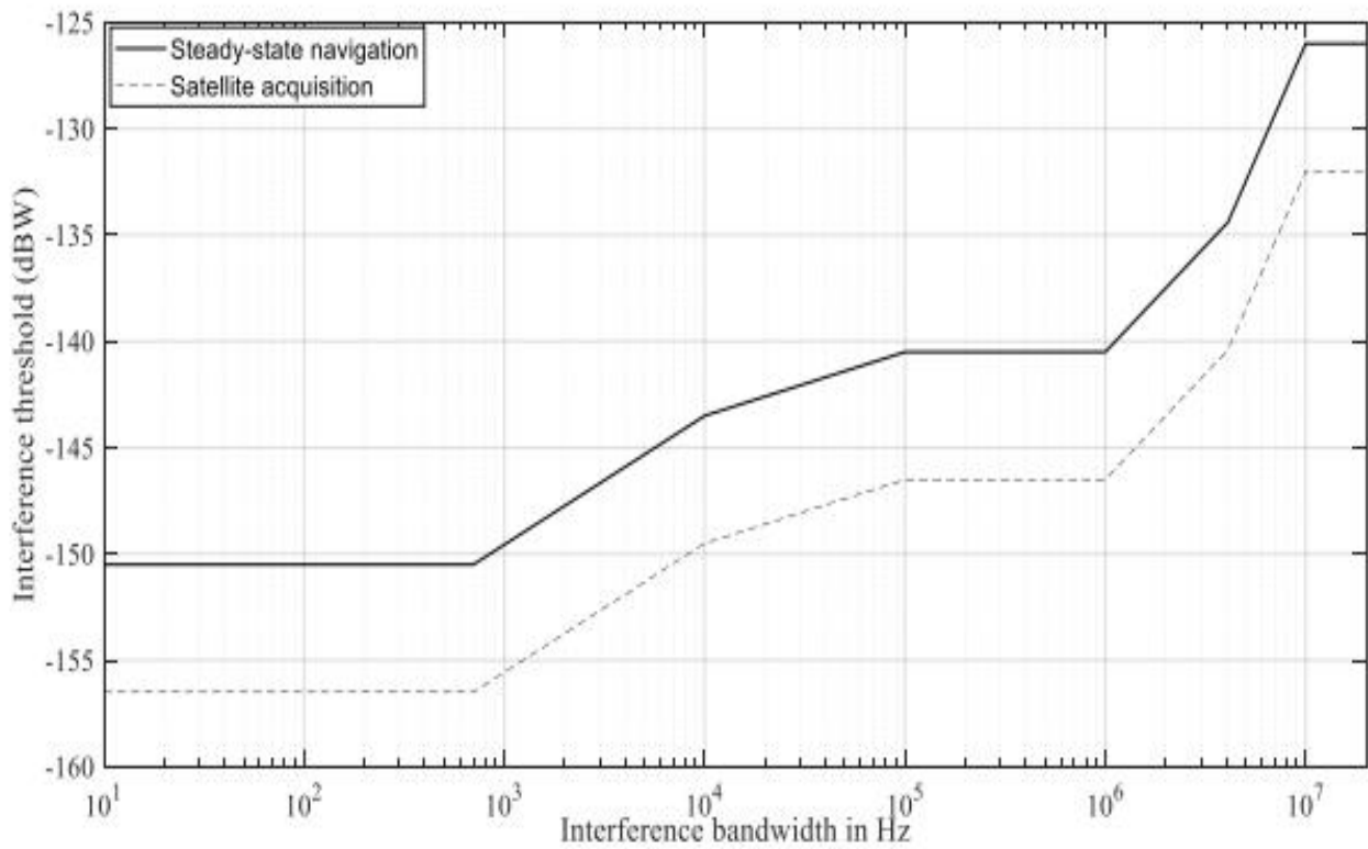
그림 B-42A. BDS B1I 수신기의 대역폭에 대한 간섭 임계값
