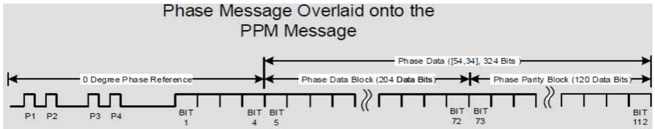
그림 3-10. 위상 오버레이 메시지 구조
