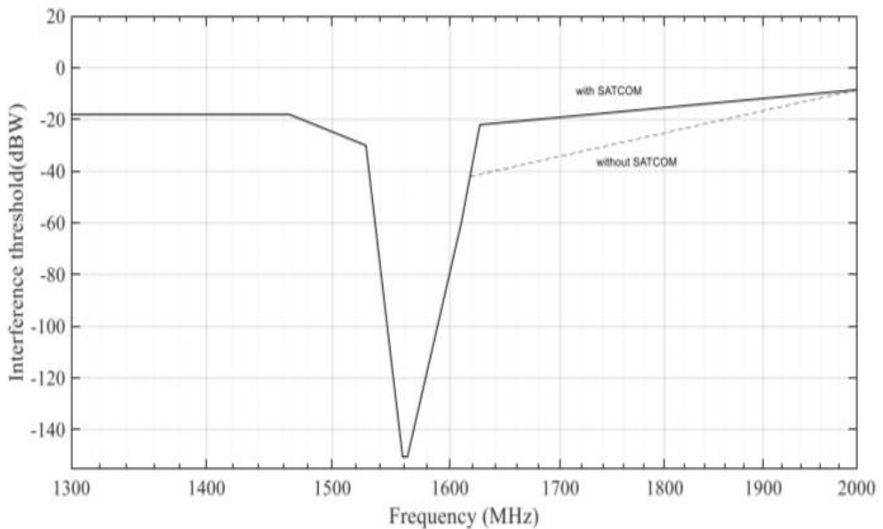
그림 B-36A. 정상상태 항법에서 BDS B1I 수신기에 대한 CW 간섭 임계값
