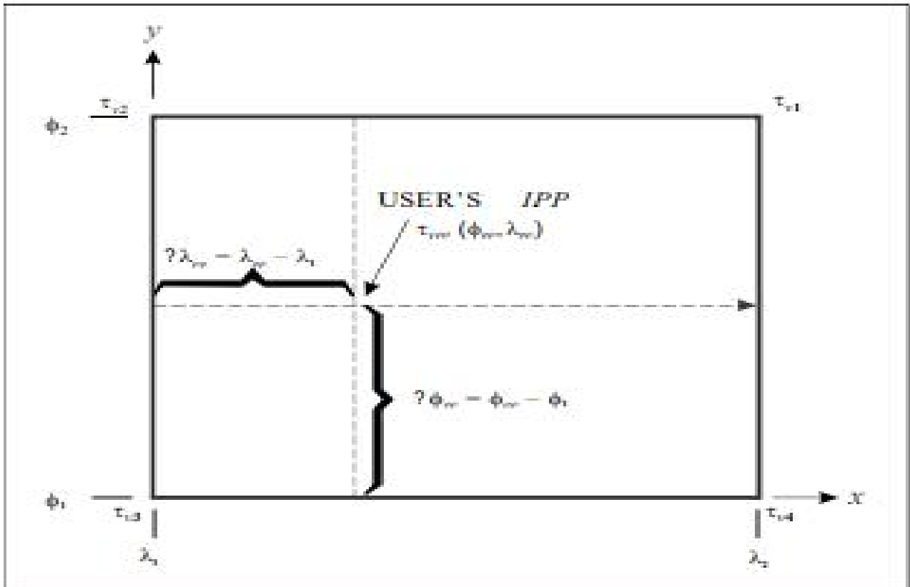
그림 B-26. IGP 번호 부여 규칙(4개의 IGP)
