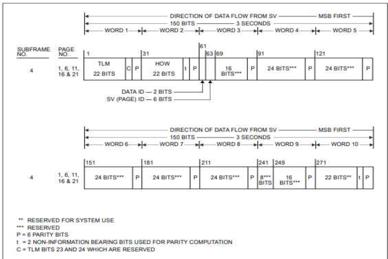
그림 B-6. 데이터 포맷(6/11)
