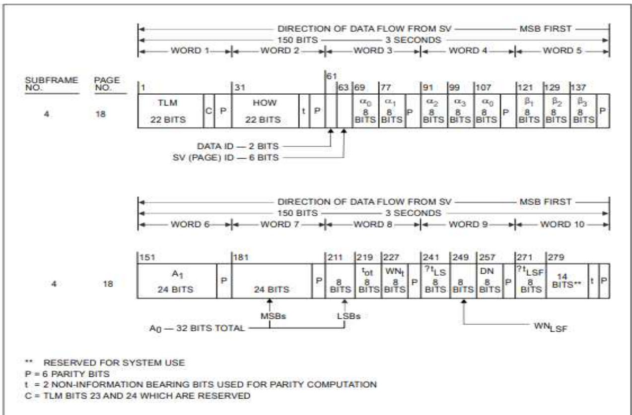
그림 B-6. 데이터 포맷(8/11)
