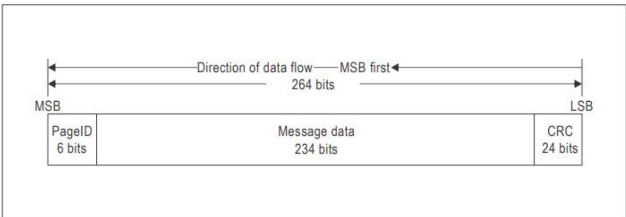
그림 B-22. B-CNAV1 서브프레임3에 대한 프레임 구조
