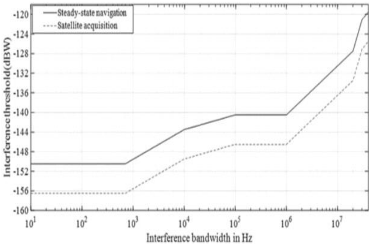
그림 B-42B. BDS B1C 수신기의 대역폭에 대한 간섭 임계값
