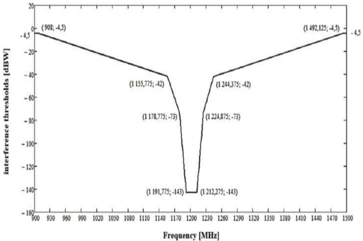
그림 B-34. 정상상태 항법에서 L3 대역의 GLONASS CDMA 신호 수신기에 대한 CW 간섭 임계값
