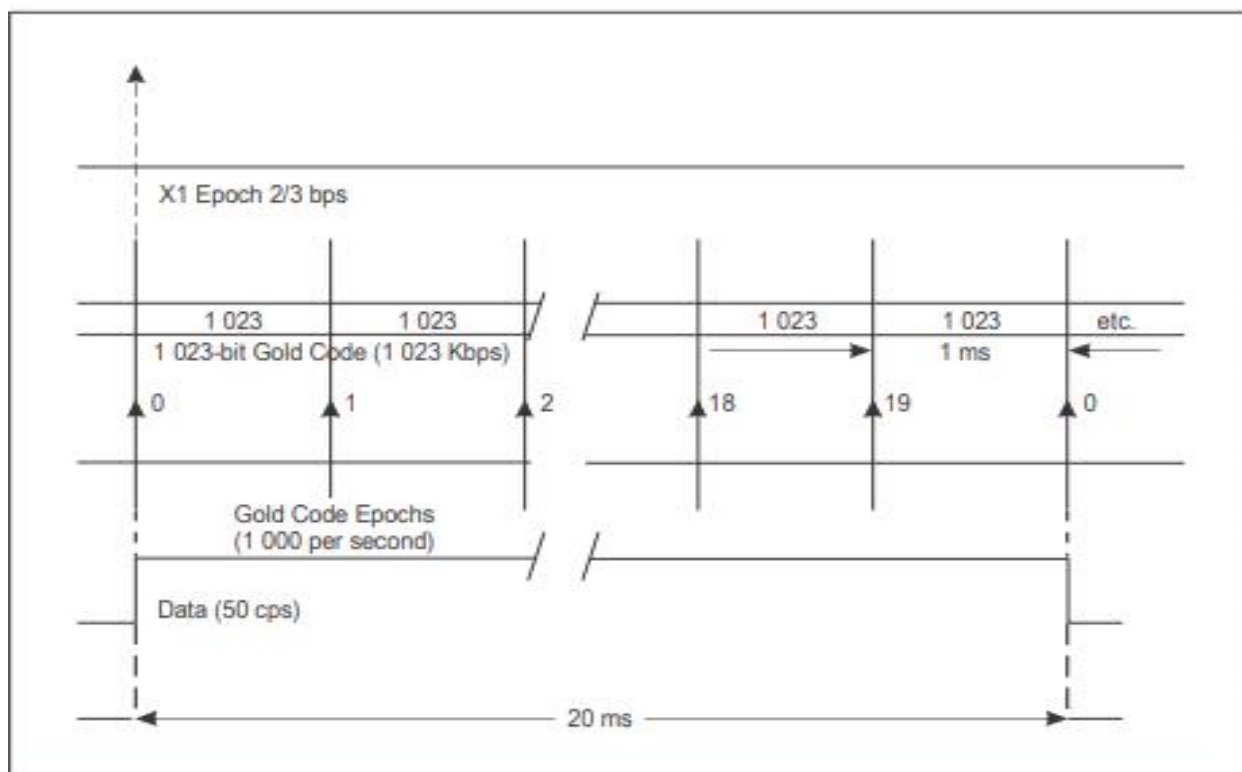
그림 B-1. C/A 코드 타이밍 관계
