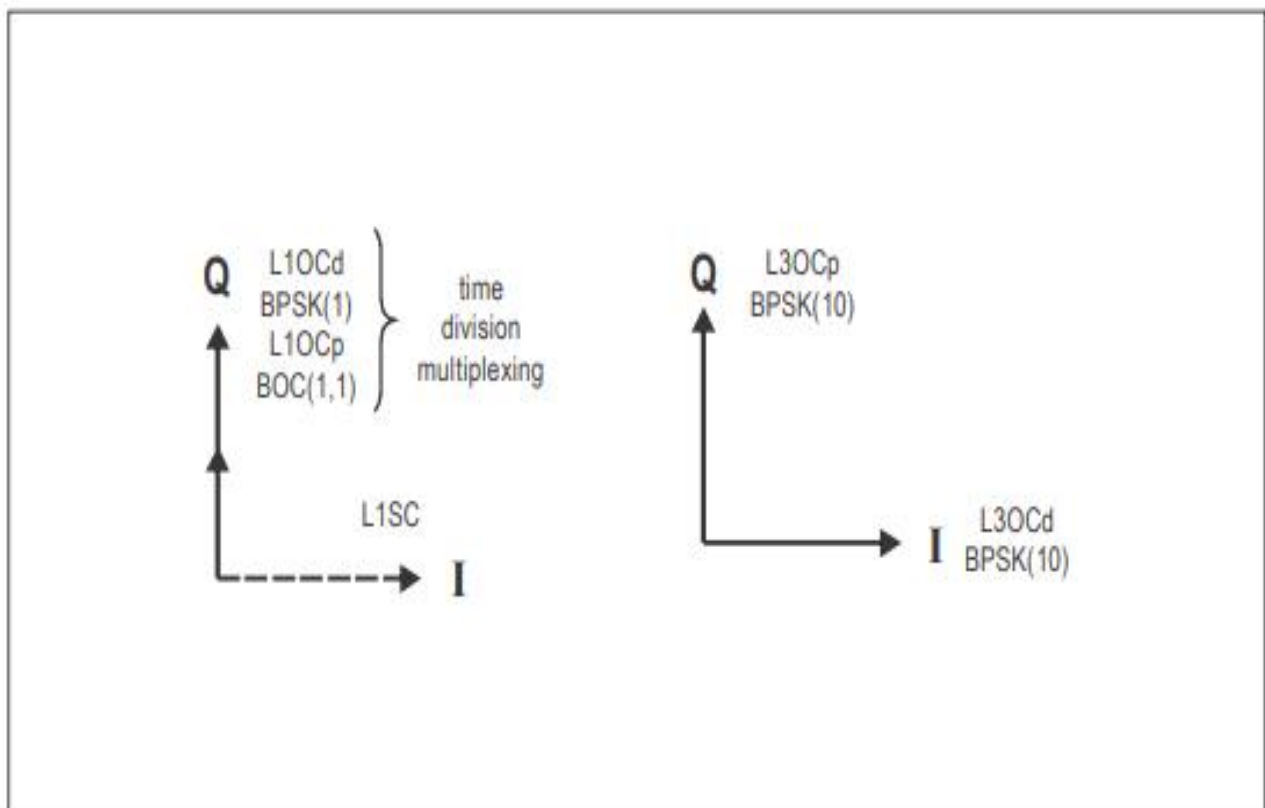
그림 B-11A. L10C와 L30C 신호 구조
