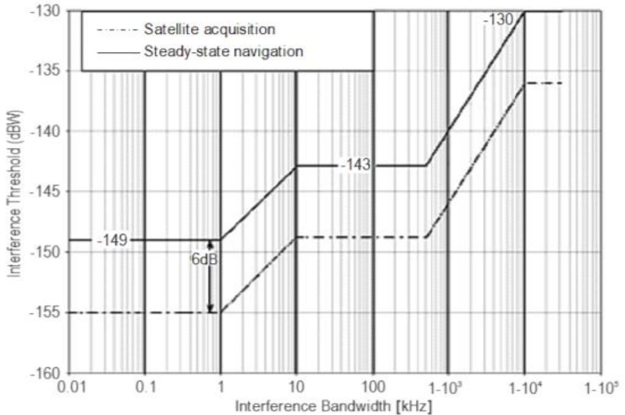
그림 B-39. L1 대역의 GLONASS CDMA 신호 수신기에 대한 간섭 임계값 대 대역폭
