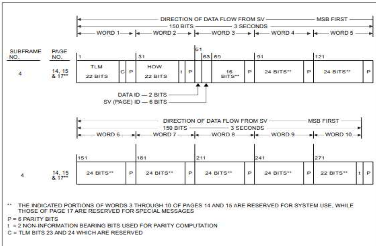
그림 B-6. 데이터 포맷(11/11)
