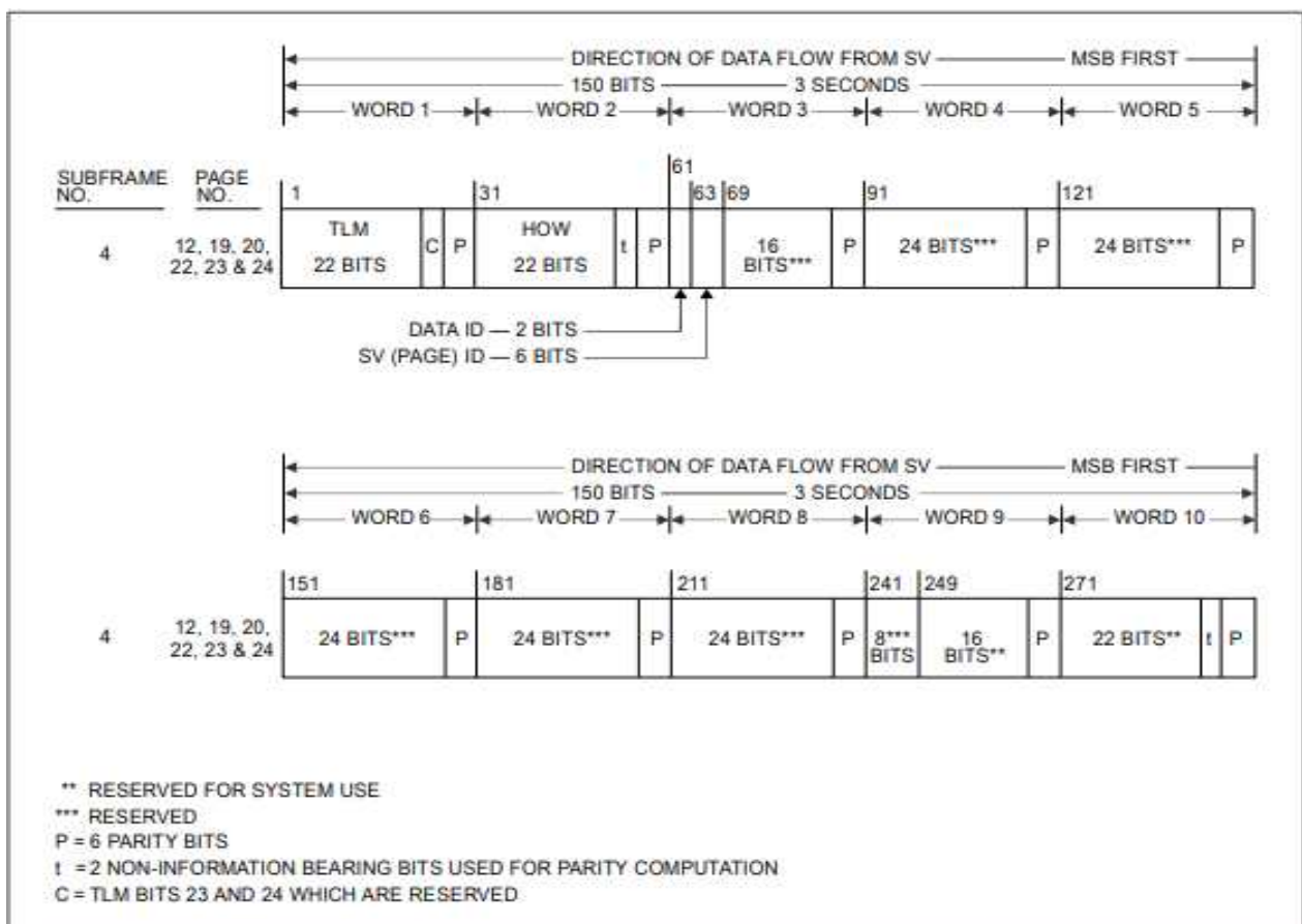
그림 B-6. 데이터 포맷(7/11)
