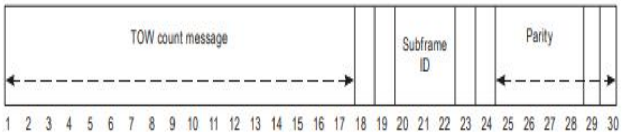
그림 B-4. HOW 포맷
