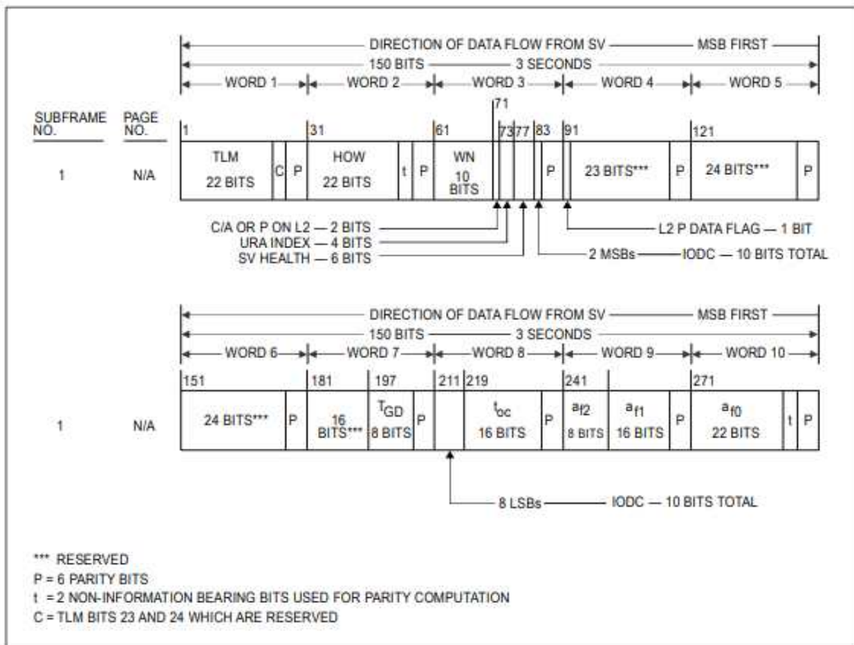
그림 B-6. 데이터 포맷(1/11)
