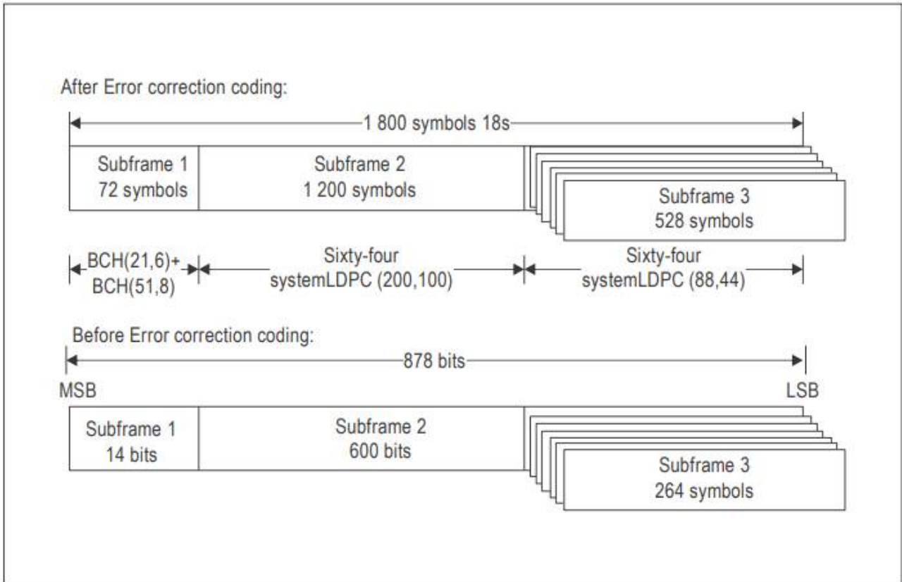
그림 B-21. B-CNAV1의 기본 프레임 구조
