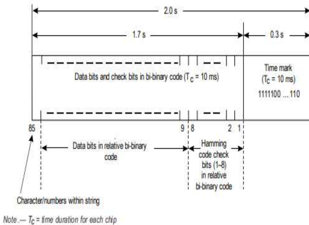
그림 B-10. 데이터 문자열 구조
