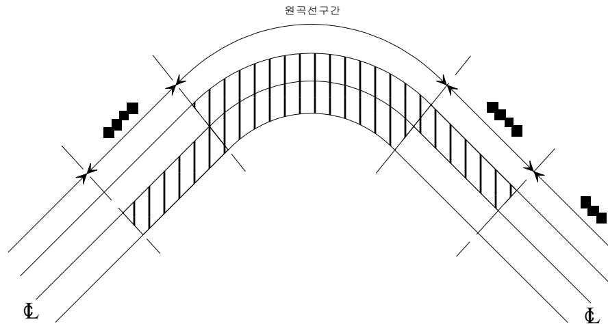
〈그림 15〉 원화구간이 있는 곡선구간에서의 미끄럼방지포장 설치
